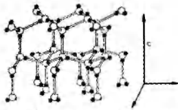
צורה 2. המבנה הגבישי של הקרח. 1. המבנה זה מתייחס רק לפיקום אטומי החמצן, המפוינים באז כבדורים נרולים ולבנים מופיע אטומי מימן; המפוינים כעגולים מפנים ושחורים איננו בטוב וביצור זה ניתנת דרישה לסידור אפשרי שלהם.
